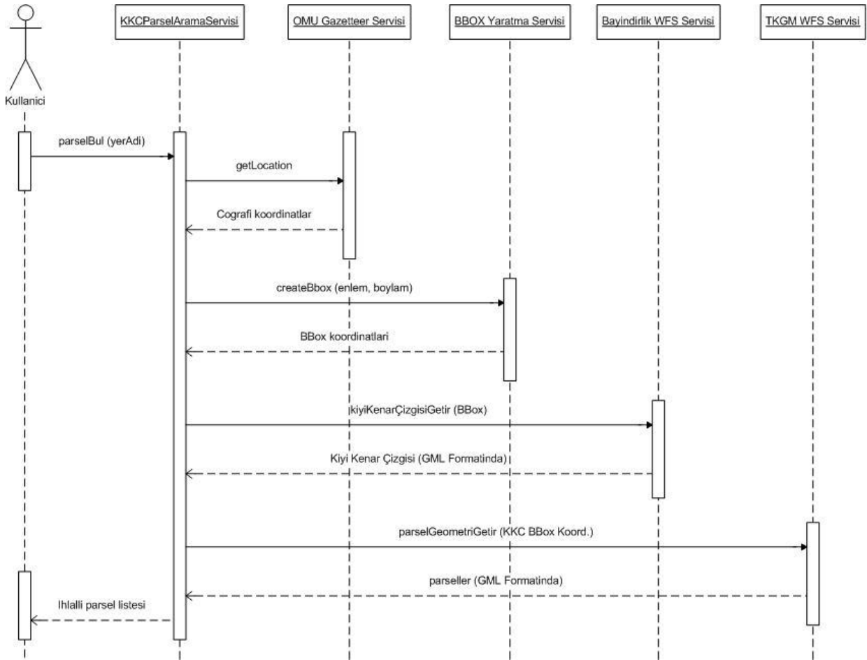
Şekil 3: KKCParselAramaServisi tarafından gerçekleştirilen uygulamanın UML ardışık iş akış (sequence) diyagramı
